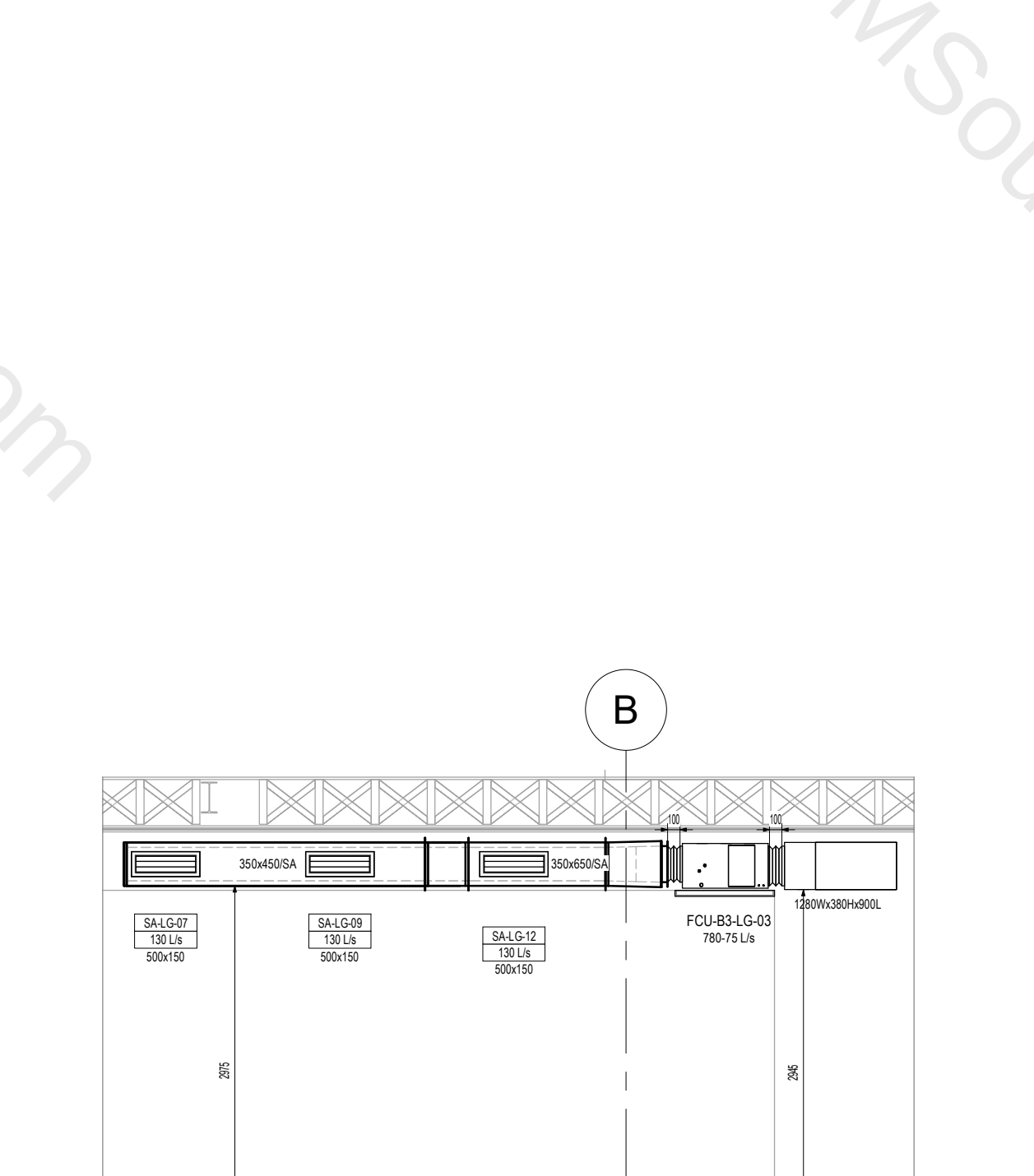
6 Section 6 1 : 50
