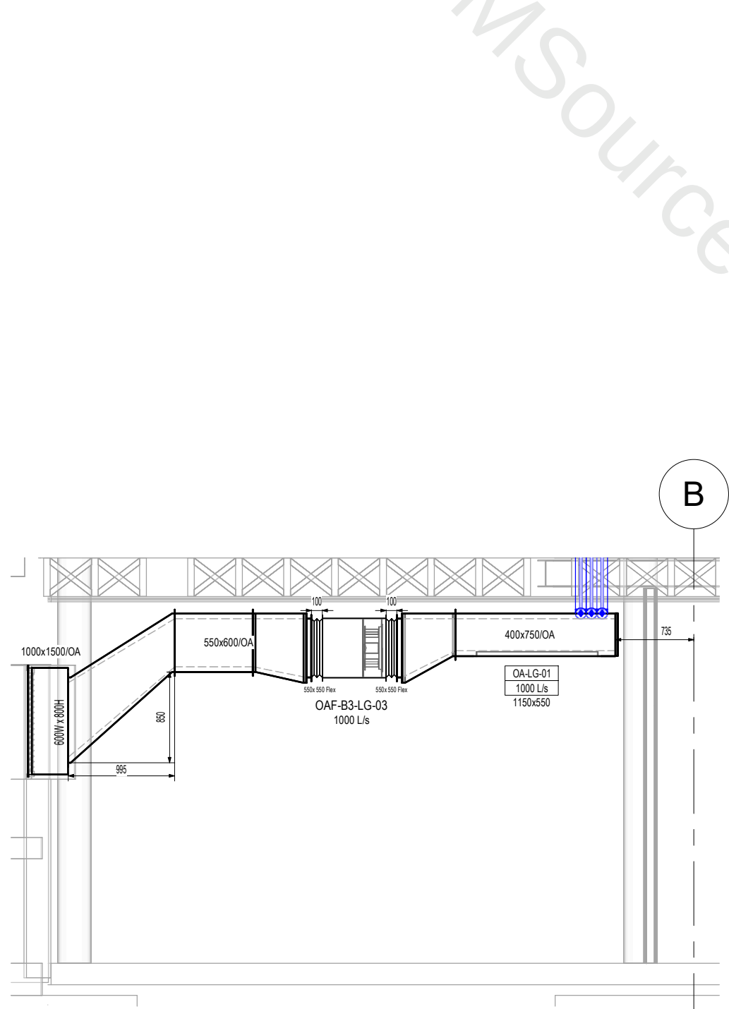
3 Section 3 1 : 50
