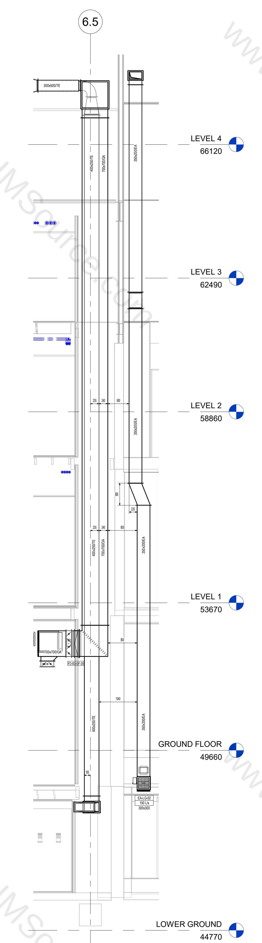
5 Section 5 1 : 50
