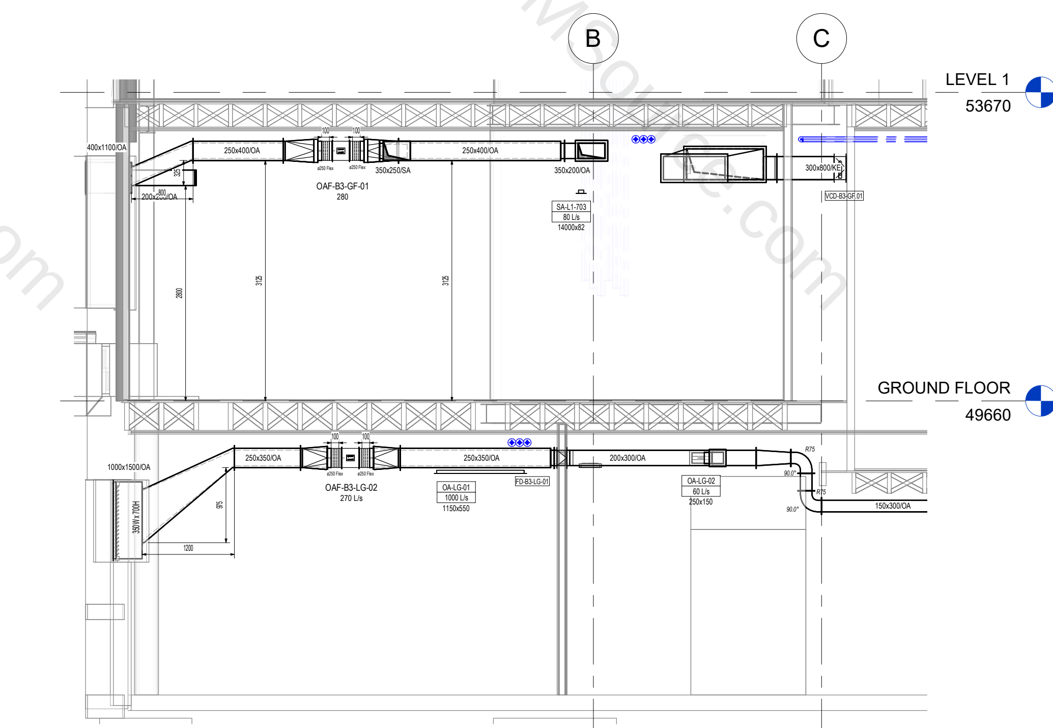
1 Section 1 1 : 50
