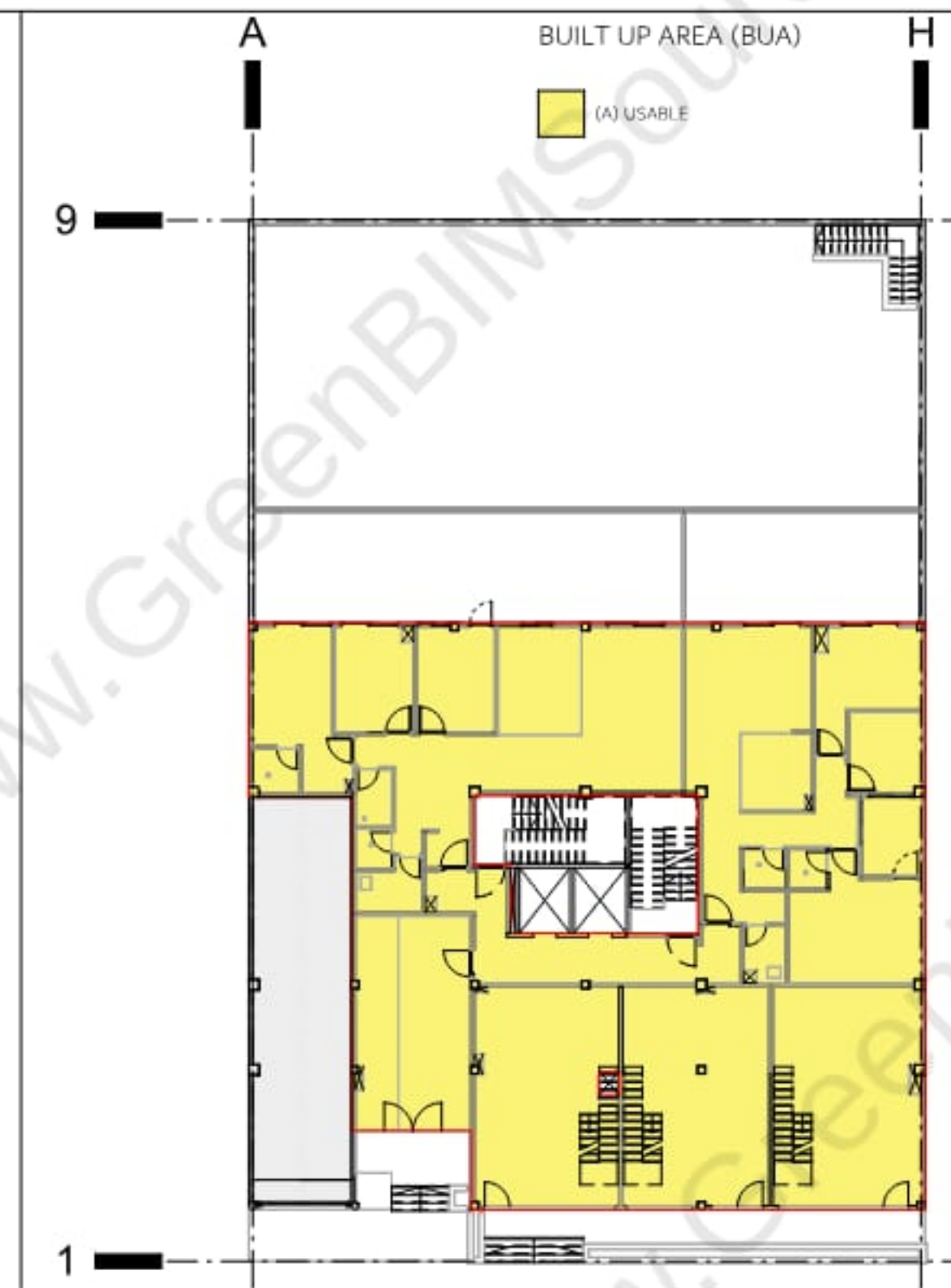
02 BUA-GROUND FLOOR (1 : 250)
